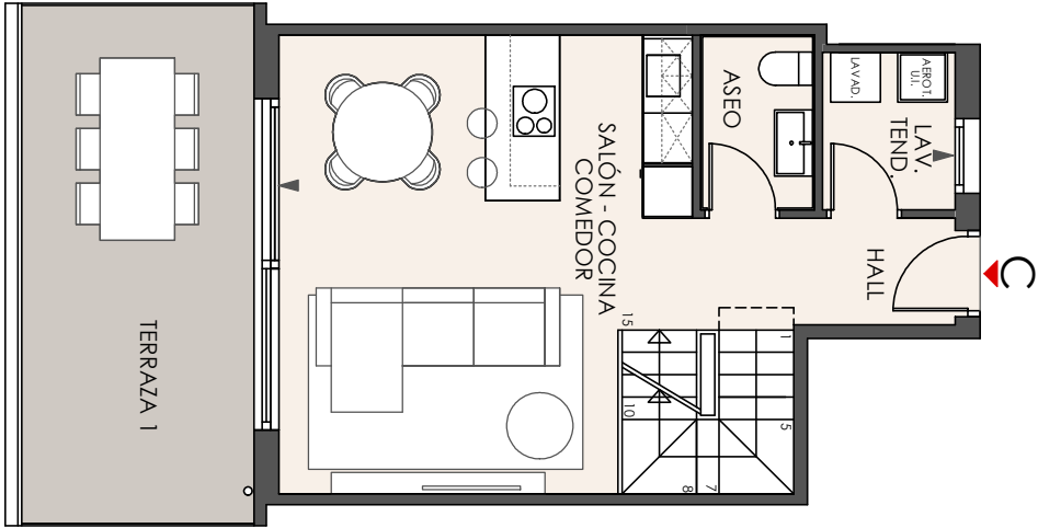
PLANTA 3ª
