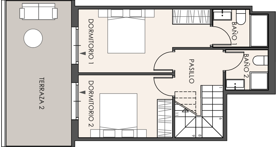
PLANTA 2ª
