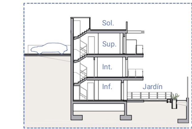
Sección / Section
