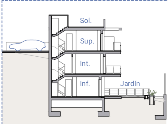
Sección / Section
